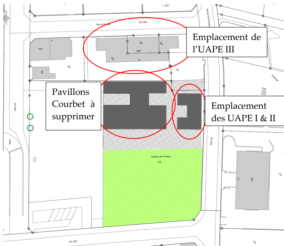
Plans d'implantation des futurs bâtiments
